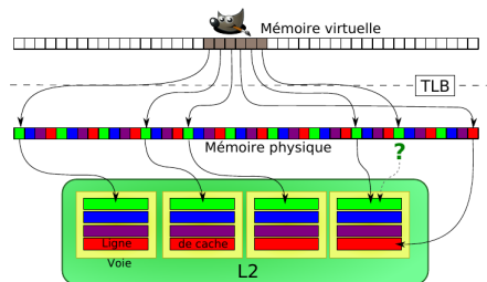
FIGURE 1 – Exemple de conflits de ligne de cache
